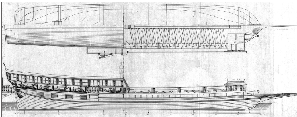
Ил. 9. 13-баночная галера «Тверь». 1767 г. Чертёж обмерный, фрагмент. Вторая половина XIX в. (ЦВММ. Сектор хранения чертежей. Инв. КП-12202/4)
