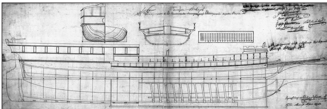
Ил. 8. Озеров М. Проект 12-баночной галеры («Тверь»). Чертёж. 1765 г. (ЦВММ. Сектор хранения чертежей. Инв. КП-12215/1)
