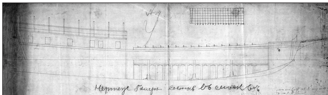
Ил. 3. Есинов. Галера «Струг московецкий», 1722 г. Чертёж обмерный. После 1749 г. (РГА ВМФ. Ф. 327. Оп. 1. Д. 4096). Публикуется впервые
