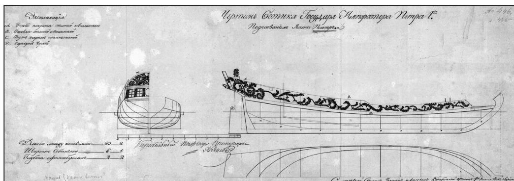
Ил. 2. Ларионов И. Плезир-яхта Петра I, 1722 г. Чертёж обмерный. Вторая половина XIX в. (ЦВММ. Сектор хранения чертежей. Инв. КП-44038/1)
