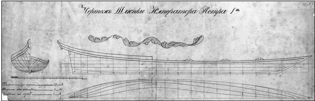
Ил. 1. Верейка Петра I, 1722 г. Чертеж обмерный. Вторая половина XIX в. (РГА ВМФ. Ф. 327. Оп. 1. Д. 5012). Публикуется впервые
