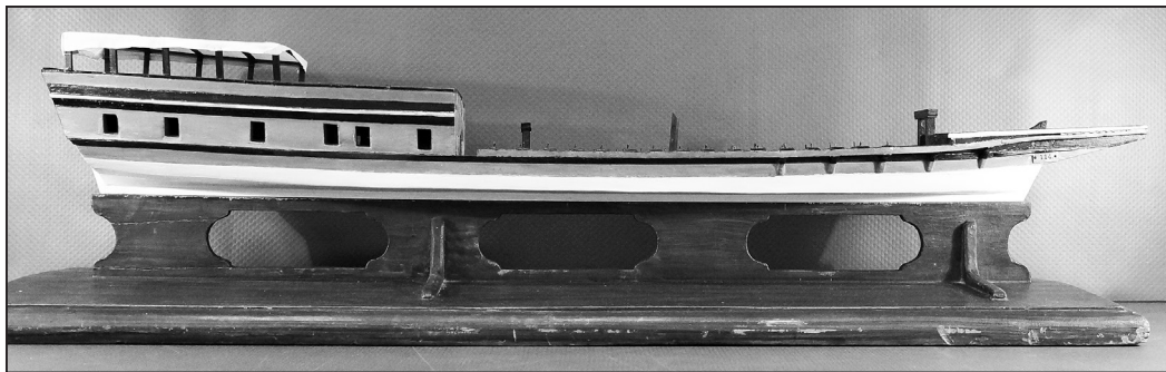
Ил. 5. Есинов. Галера «Струг москворецкий». 1722 г. Модель. После 1749 г. (ЦВММ. Инв. КП-176)
