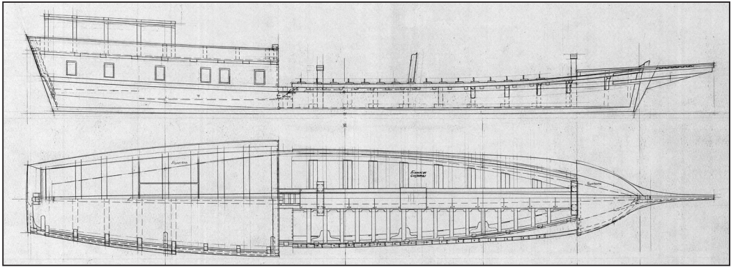
Ил. 7. Иванов А.В. Модель галеры «Струг москворецкий». Чертёж обмерный, фрагмент (Инв. КП-176. 2013). (Собрание автора)
